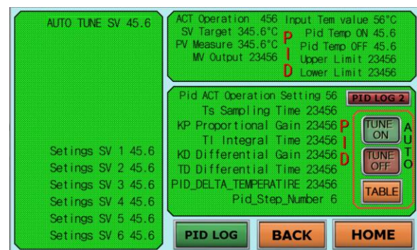
Fig. 7. PID control.
