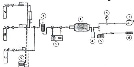
Fig.1. The sintering system;
